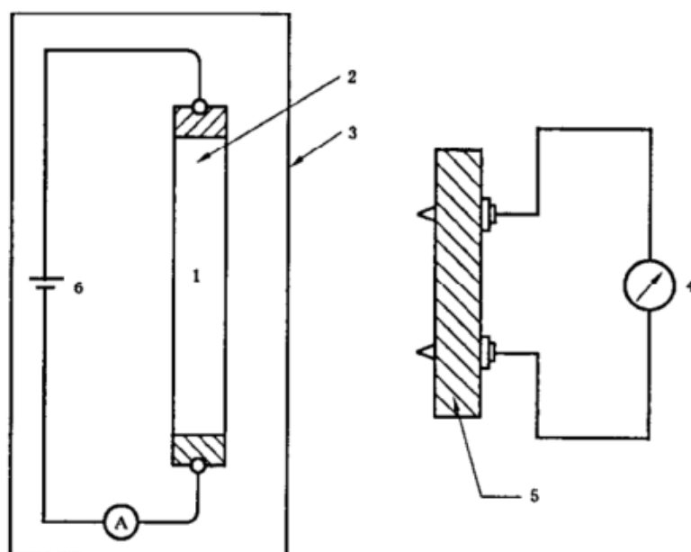
1—试样;2—电流电极;3—绝缘垫,电阻至少 10^{12} \Omega ;4—电位计(静电计);5—电压电极;6—可调式直流电压
